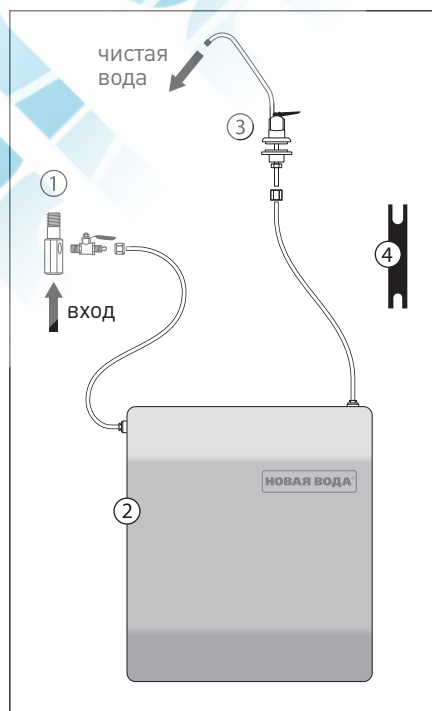
Схема подключения фильтра Expert.
