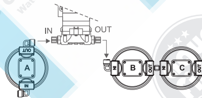
ВИД КОРПУСОВ ПРЕФИЛЬТРОВ СВЕРХУ версия без насоса
