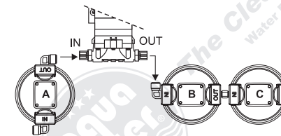
WIDOK KORPUSÓW FILTRÓW WSTĘPNYCH Z GÓRY wersja z pompą
